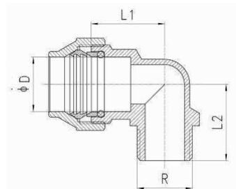
Codo 90° Macho PE/M Male elbow 90° PE/M
