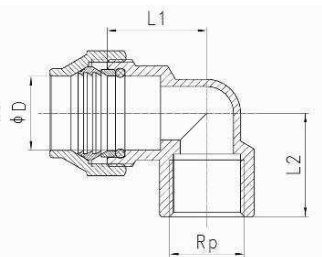
Codo 90° Hembra PE/M Female elbow 90° PE/F
