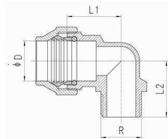
Codo 90º Macho PE/M Male elbow 90º PE/M
