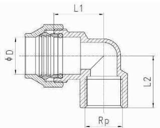
Codo 90º Hembra PE/M Female elbow 90º PE/F
